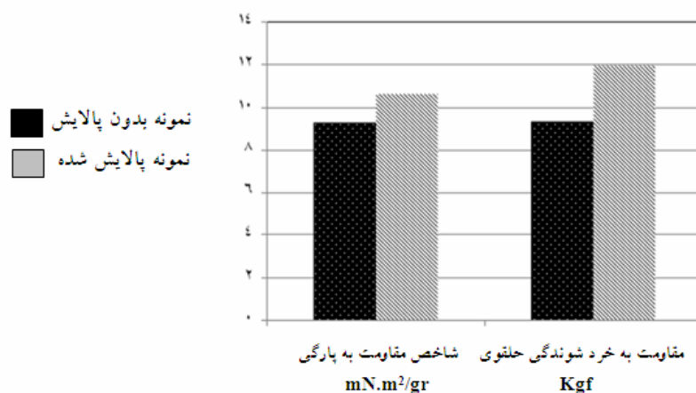
شکل ۶- مقایسه شاخص مقاومت به پارگی و مقاوت به خردشوندگی حلقوی (RCT) خمیر کاغذ شاهد و پالایش شده
